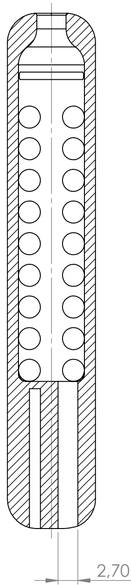
SECTION A-A
